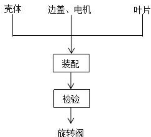
图 2-4 旋转阀生产工艺流程及产污环节图
