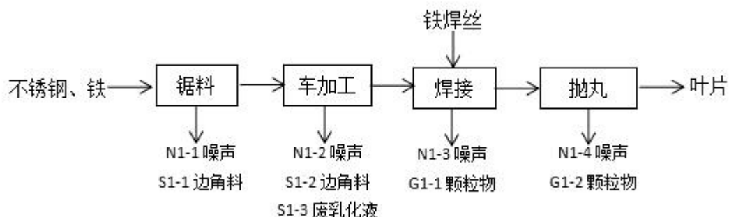
图 2-3 叶片生产工艺流程及产污环节图
